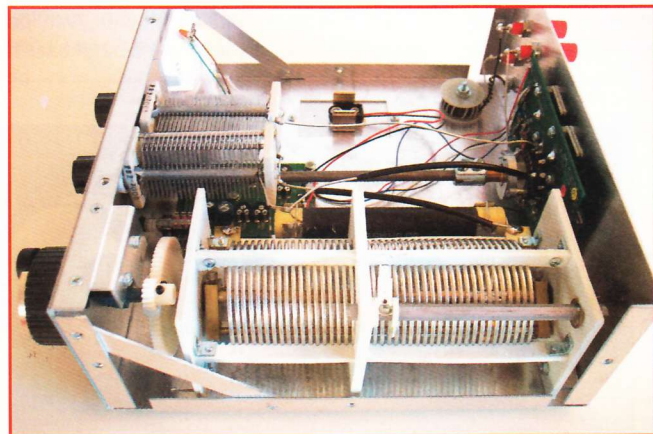
MFJ-969 inwendig.
